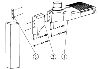
Pole Carré Bras Droit
